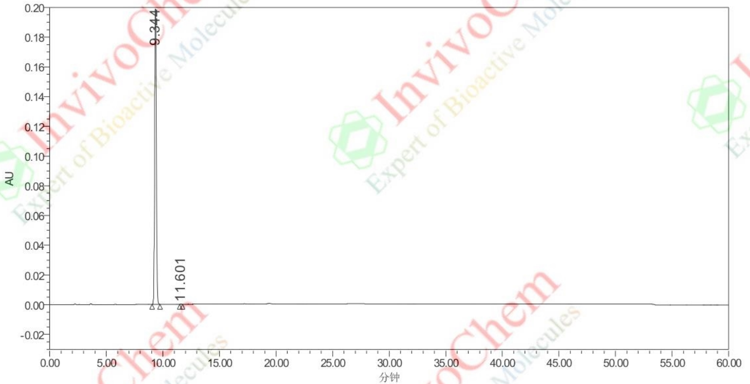
色谱峰结果
