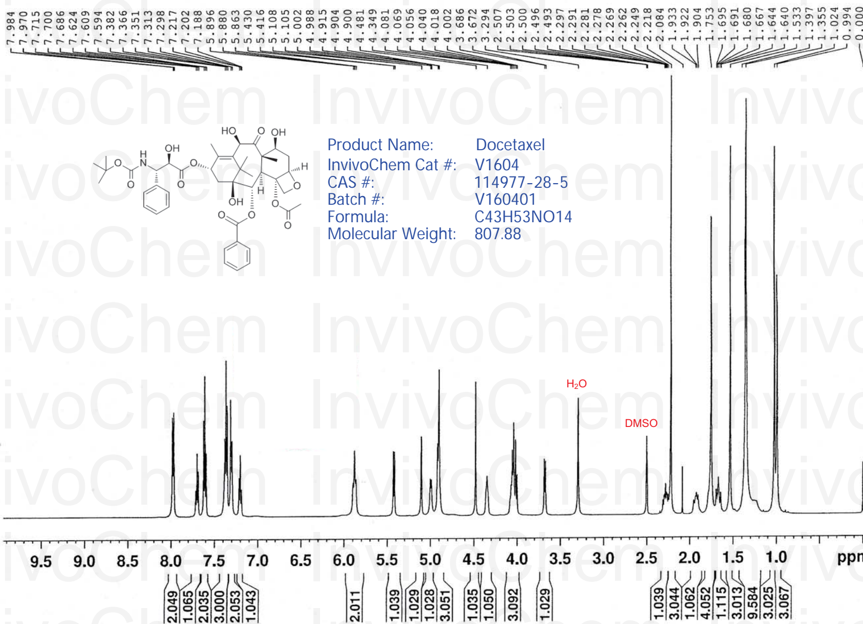
图 5a 多西他塞样品 (批号: 120825) 的氢谱
