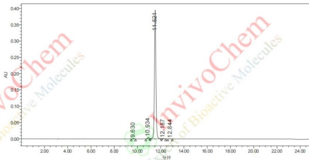
色谱峰结果
